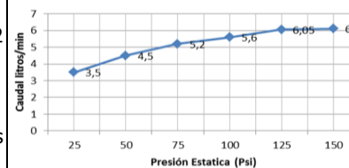
Consumo con Aireador Inteligente
