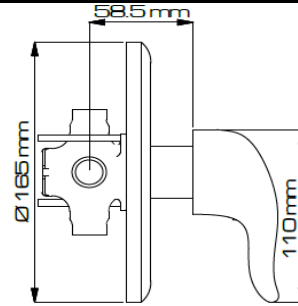
Vista Lateral Ensamble
