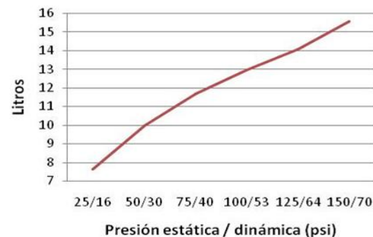
Consumo sin regadera (L/min)
