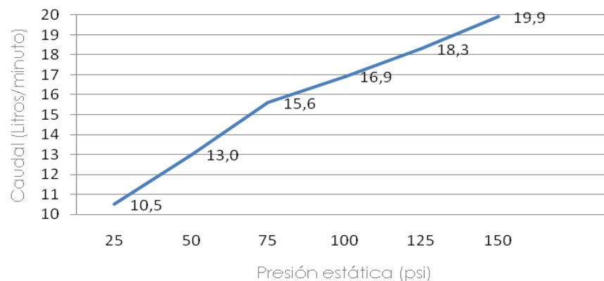
Consumo Monomando
